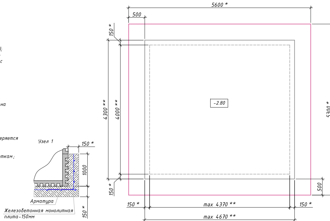
План котлована с плитой
