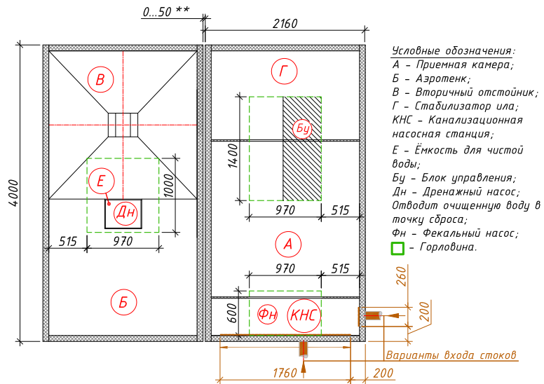
Схема станции
